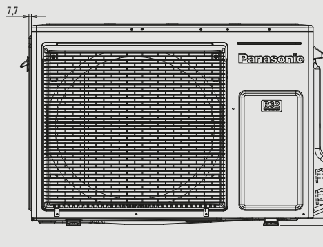
Frontansicht
