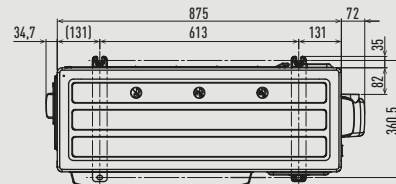
Draufsicht
