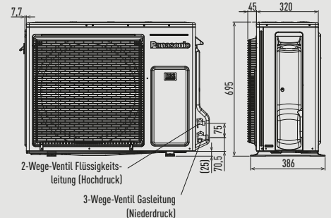
Frontansicht
